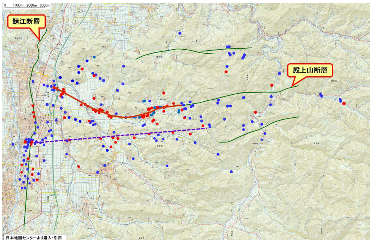
図 14. 地下水中の炭酸水素イオン濃度またはフッ化物イオン濃度が高い地点と破碎帯（断層）の位置
