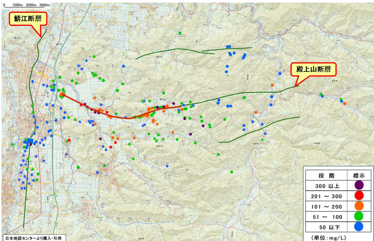
図 12. 地下水中の炭酸水素イオン濃度の分布
