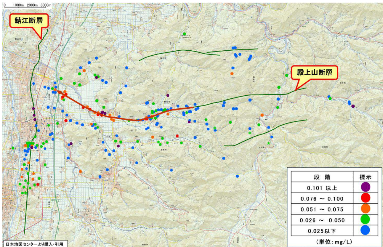
図 13. 地下水中のフッ化物イオン濃度の分布
